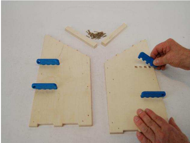
1. Stecken Sie blauen Scharniere in die entsprechenden Aussparungen der Seitenteile
