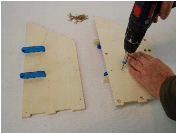
3. So können Sie die Scharniere bequem von der anderen Seite verschrauben, ohne dass rausrutschen können.
