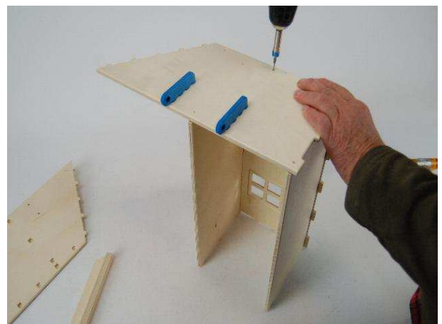
6. Stecken Sie ein passendes Seitenteil auf Rückwand und Böden und verschrauben beides
