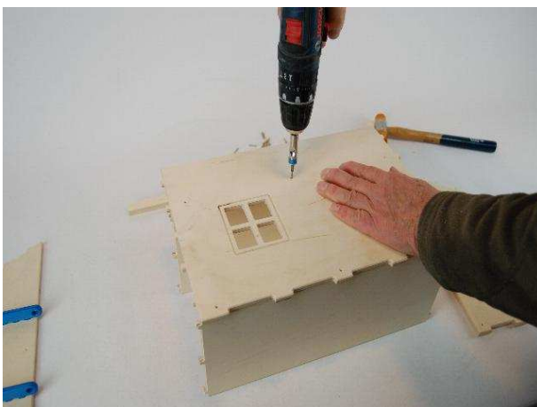
5. Drehen Sie alles vorsichtig um und verschrauben Böden und Rückwand mit 6 Schrauben
