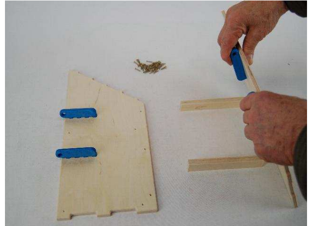
2. Benutzen Sie die beigelegten Leisten zum Unterlegen
